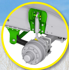
Hydro-Tridem Federung
